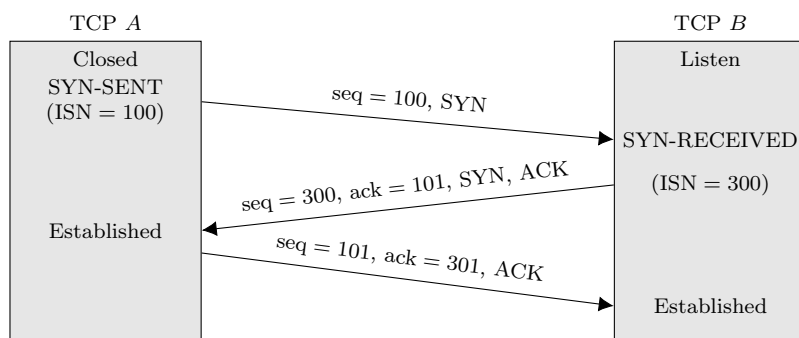
Figura 3.1: Establecimiento de conexión TCP sin incidencias.
