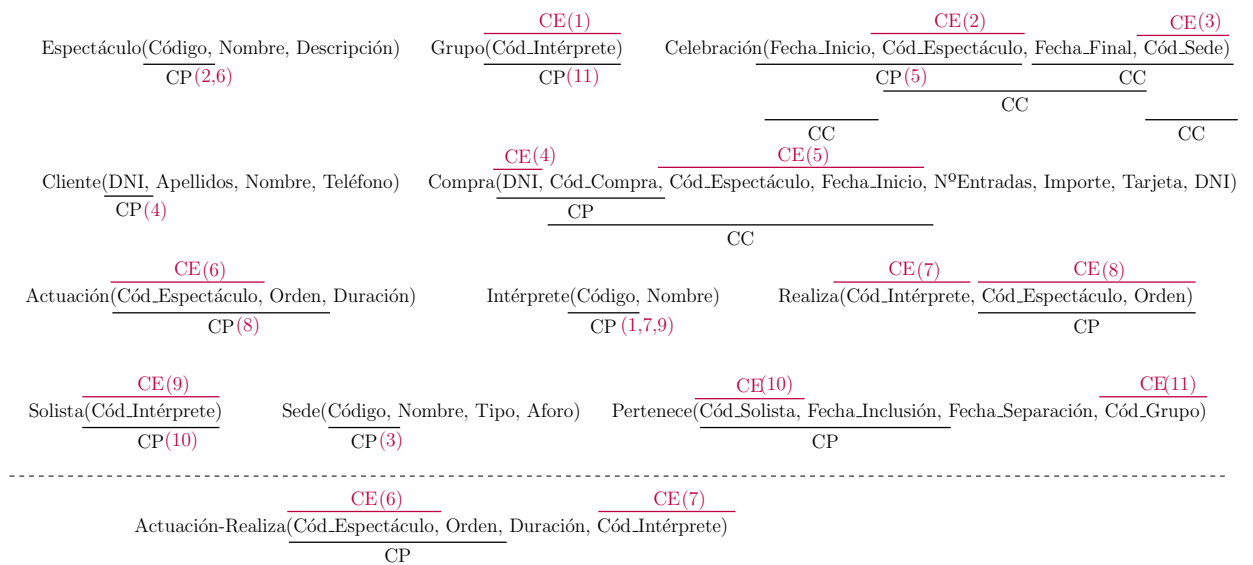
Figura 2: Esquema Relacional.
