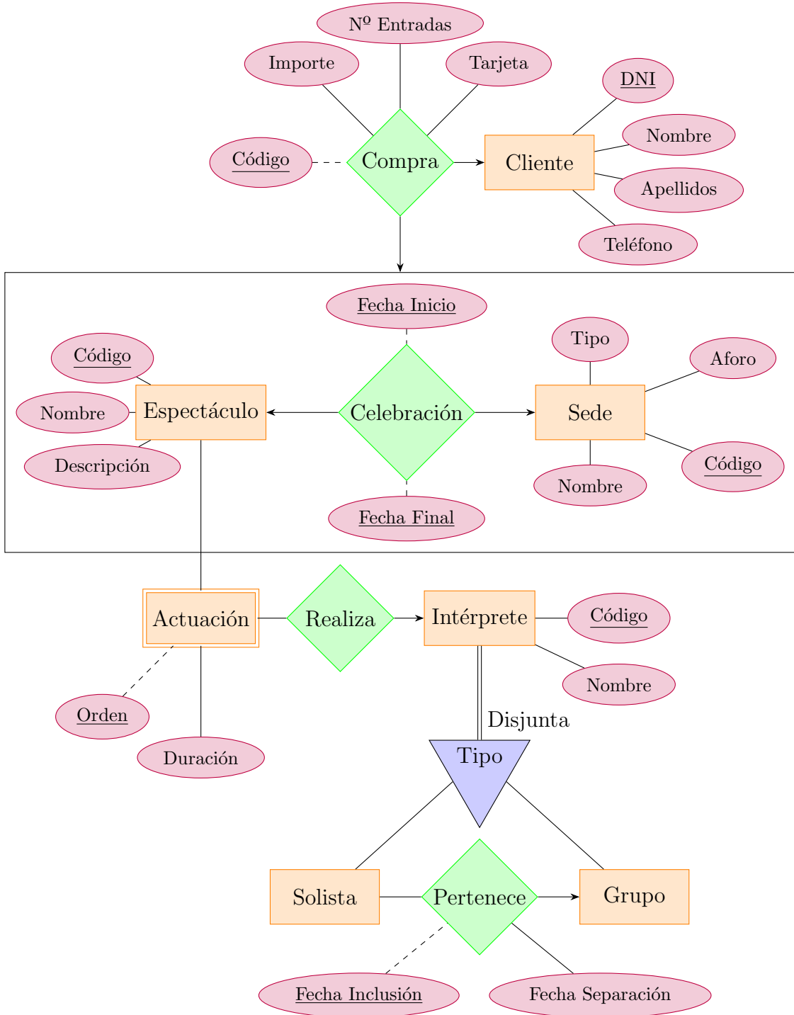
Figura 1: Esquema Entidad/Relación.
